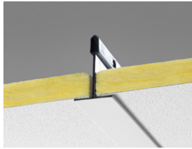
Detalhe do sistema Gedina A
