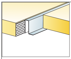
Konstrukcija kopā ar padziļinājuma profilu /p>
