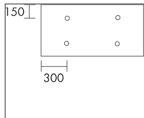
Skrūves ar izmēru 1200 x 600 novietojums
