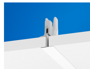
Hlavní profil Connect T24 C4 Connect Hygiene klipem
