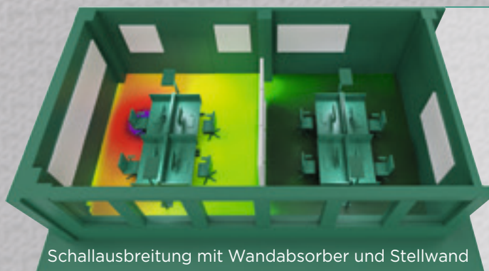
Schallausbreitung mit Wandabsorber
