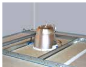
Montážní pružina (2 ramena) instalována pomocí Connect přemostění
