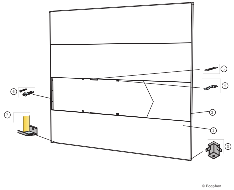
M592 Diagrama de instalación (M592) para Ecophon Akusto Wall C instalado horizontalmente con Connect Marco Thinline
