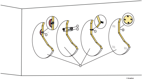
M372 Diagrama de instalación (M372) de Ecophon Akusto One
