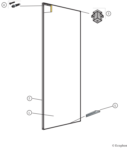
M593 Diagrama de instalación (M593) para instalación vertical de panel Ecophon Akusto Wall A con Connect Marco Thinline.
