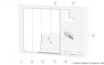
M609 Diagrama de instalación (M609) para Ecophon Akusto Wall C instalado verticalmente con Connect perfil Thinline.
