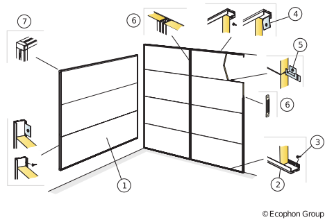
M355 Diagrama de instalación (M355) para Ecophon Akusto Wall C instalacion horizontal
