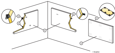
M371 Diagrama de instalación (M371) de Ecophon Akusto One
