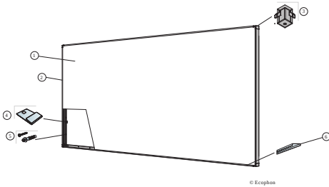
M595 Diagrama de instalación (M595) para instalación horizontal de Ecophon Akusto Wall A con Connect Marco Thinline.
