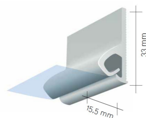
Clipso P-CW profiili seinäsennuksiin (taulut) ja alaslasketulle katolle
