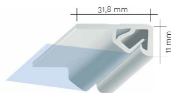
Clipso P-CC profiili reunasta reunaan ulottuviin seinä- ja kattoasennuksiin
