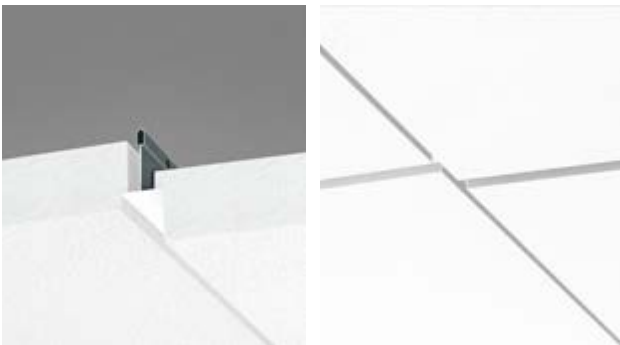
Eritasoinen pykäläreuna, jossa levy asettuu vinoon, avattavissa (Focus)
