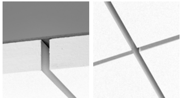
Suorareunainen liima-asennus avosaumoin, ei avattavissa
