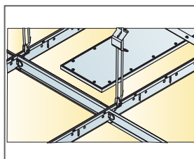
Line lp armaturhus vilar på tvärprofilen
