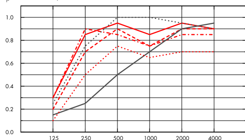
\alpha_{pr} Coeficiente práctico de absorción de sonido
