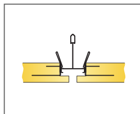
Overgang tussen twee niet dragende zijdes met Kantsclip
