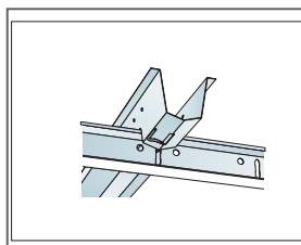
Spojení profilů pomocí Connect závěšky pro vymezořač
