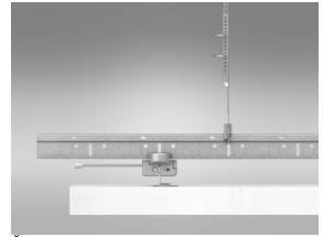
Řez systémem Solo Matrix
