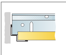
Taisns griezumums, panelis atbalstīts uz ēnu profila
